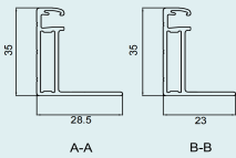
A-A
